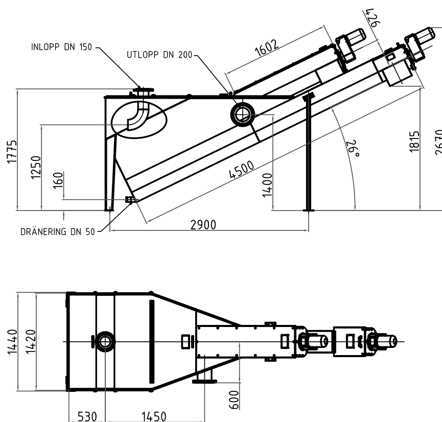
Standardritning DA 320.
