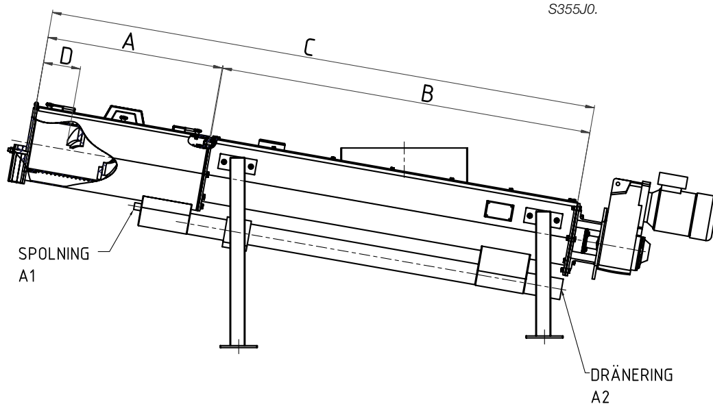
Invändig vy över pressrör i Wedge Weir och spiral i svart material S355J0.
